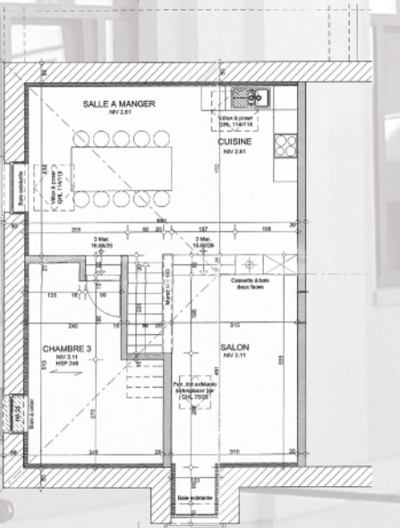
PLAN ETAGE
