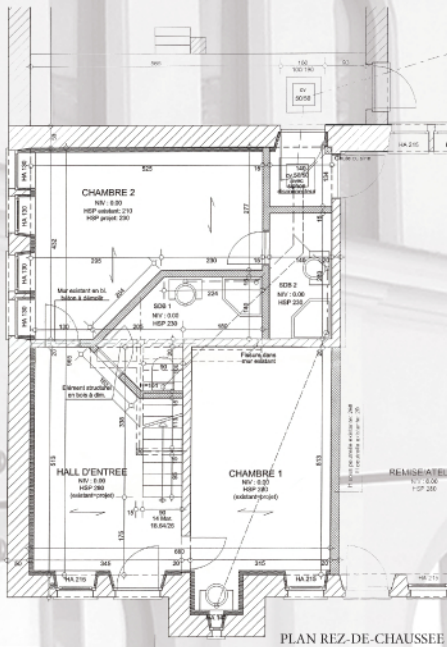
PLAN REZ-DE-CHAUSSEE
